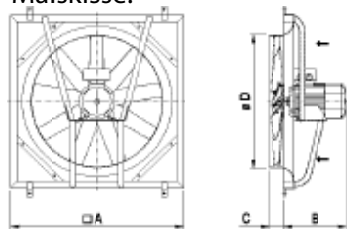
Målsskisse:
