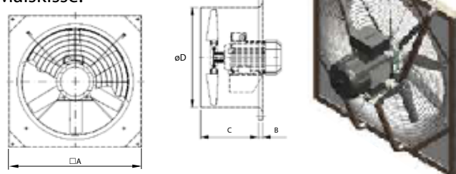
Målsskisse:
