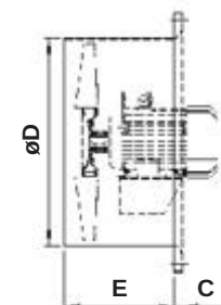
Målsskisse BP 25R - BP 35
