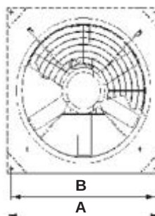
Målsskisse BP 25R - BP 35
