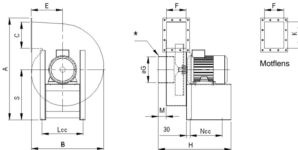
Målskisse
